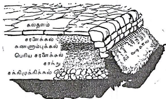
உரோமர் சாலை அமைத்த விதம்
